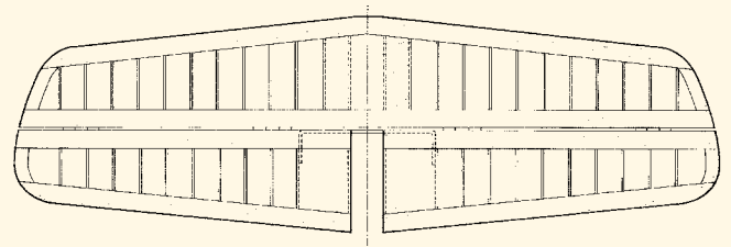
Ritning finns i A4-format i LINA 91.1 och MFN 66.5-6. Den som är intresserad av att bygga en Silverbird kan höra av sig till Ove och få ritningsfiler mejlade.
